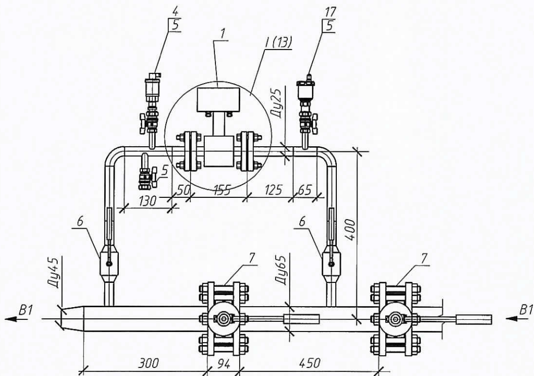
Аксонетрическая схема В1
