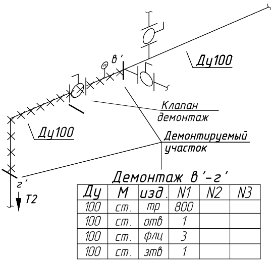
Узел ввода T2 в ТЦ №2 до монтажа УЧ
