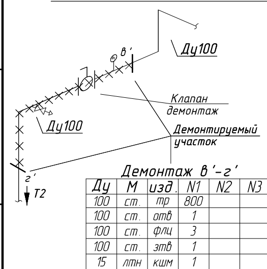
Узел ввода T2 в ТЦ №4 до монтажа УЧ
