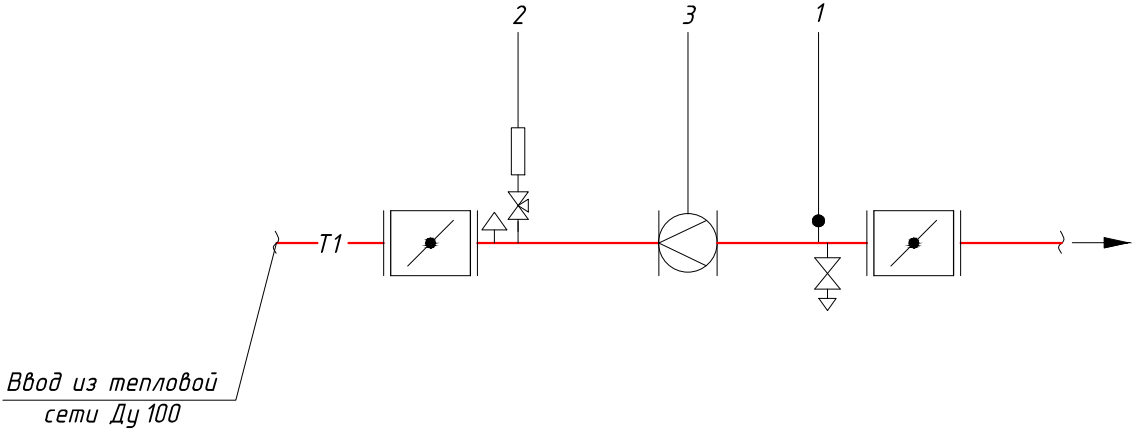
УУТЗ-4
