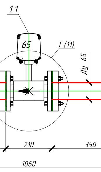
T2-2 Вид В (Масштаб 1:10 А3)
