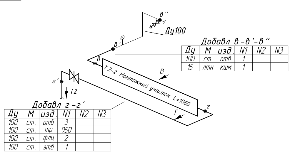
Узел ввода T2 в ТЦ №4 после монтажа УЧ
