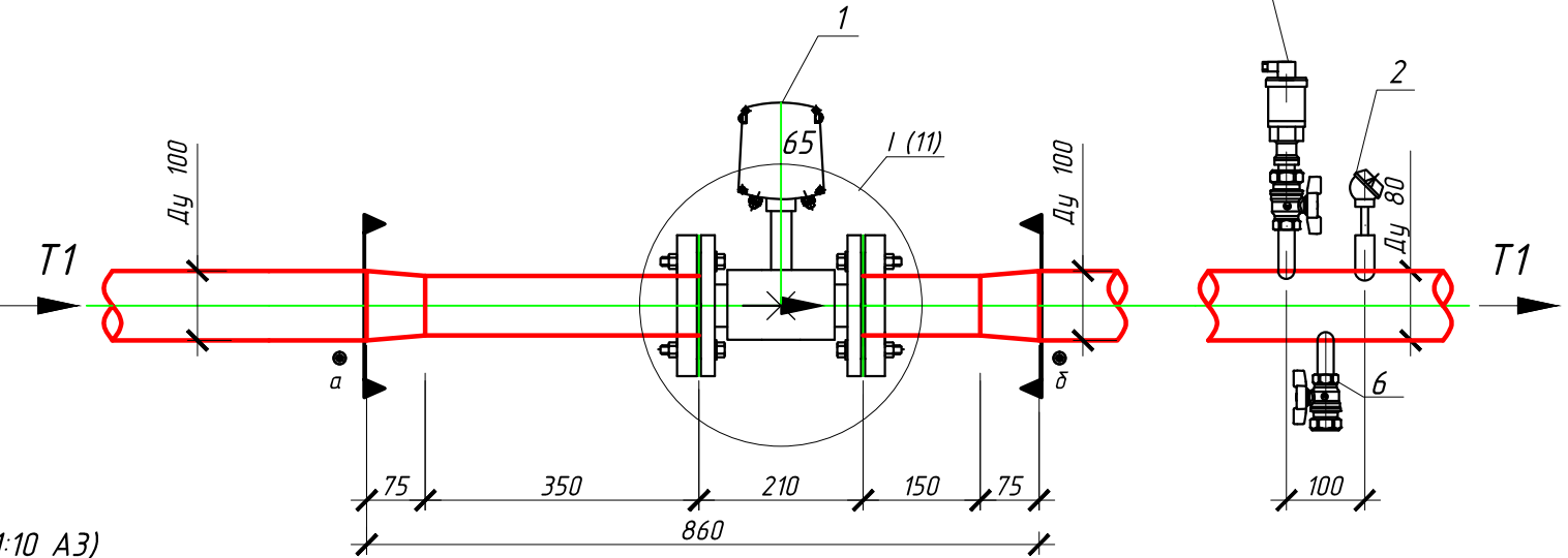
T2-2 Вид В (Масштаб 1:10 А3)
