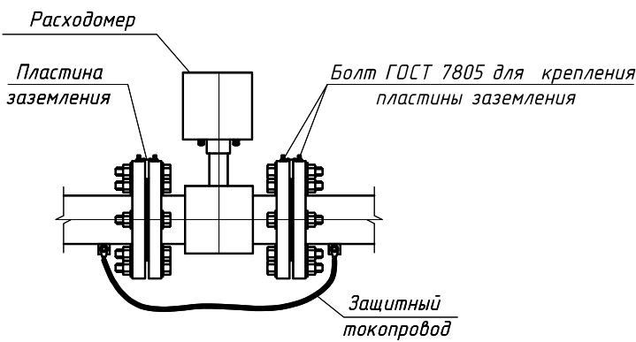
Фрагмент I
