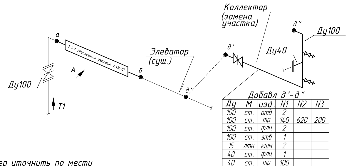
Узел ввода T1 в ТЦ №1 после монтажа УЧ
