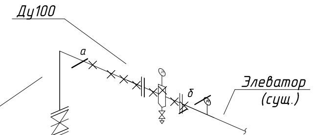
Узел ввода T1 в ТЦ №1 до монтажа УЧ
