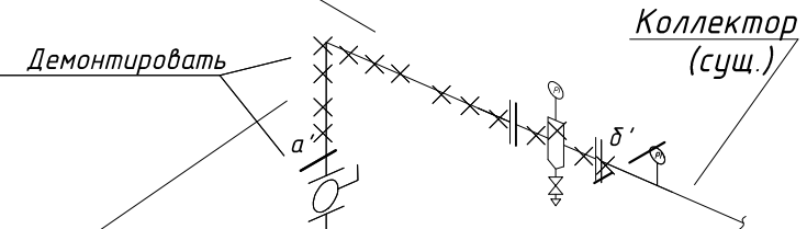
Демонтаж а'-б'
