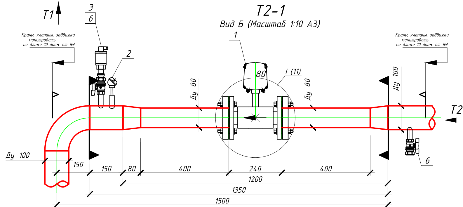
Узел ввода T2 в ТЦ №1 после монтажа УЧ
