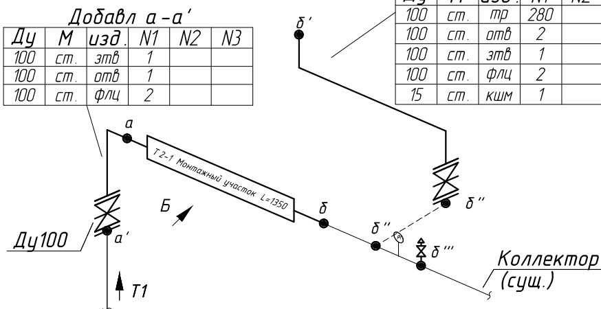
Узел ввода T2 в ТЦ №1 после монтажа УЧ
