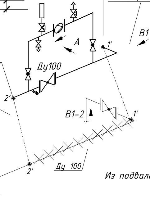
Точка врезки 1
