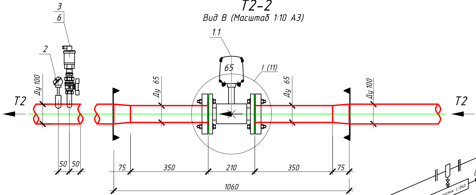
Вид Г (Масштаб 1:10 А3)
