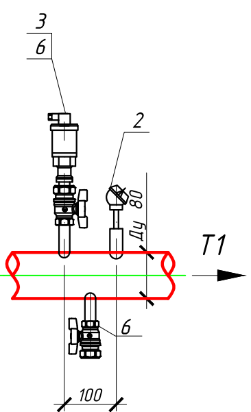
Вид Б (Масштаб 1:10 А3)
