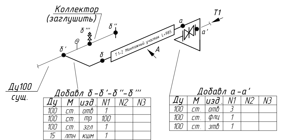
Узел ввода T1 в ТЦ №3 после монтажа УЧ
