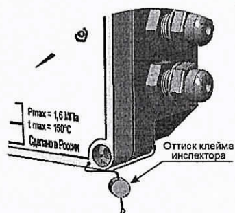
Схема пломбирования МФ
