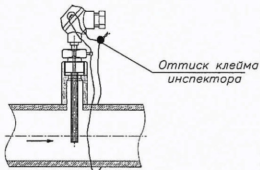
Схема пломбирования термопреобразователя
