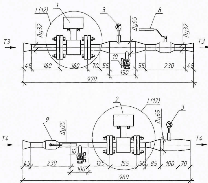
Аксонетрическая схема ТЗ
