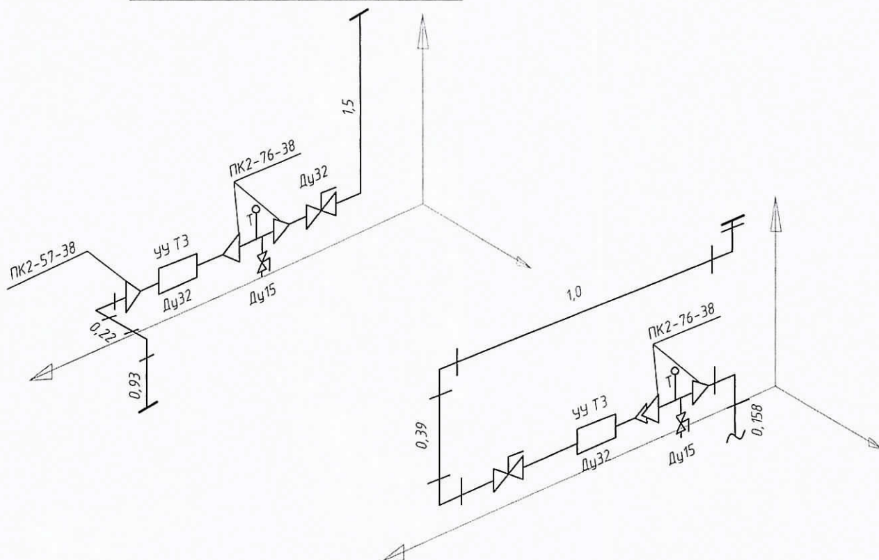
Аксонетрическая схема ТЗ
