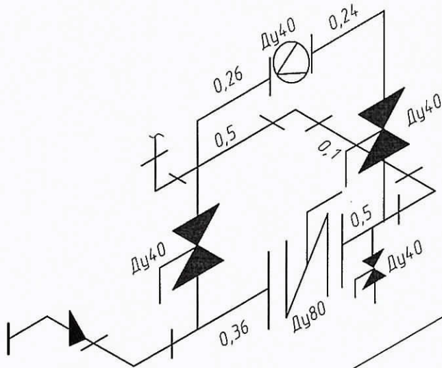
Аксонметрическая схема В1
