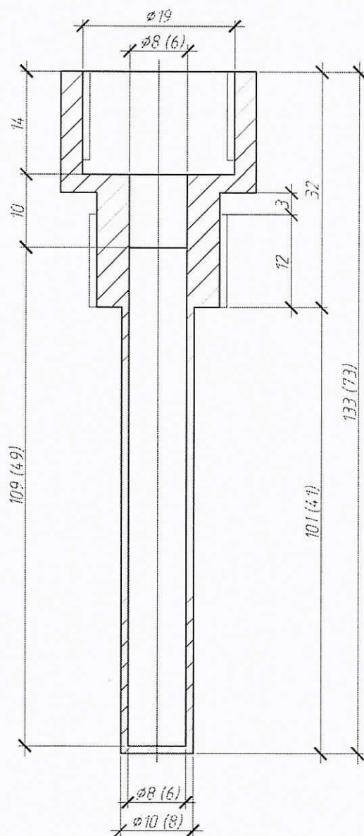
Гильза термопреобразователя сопротивления
