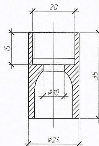
Бобышка термопреобразователя сопротивления
