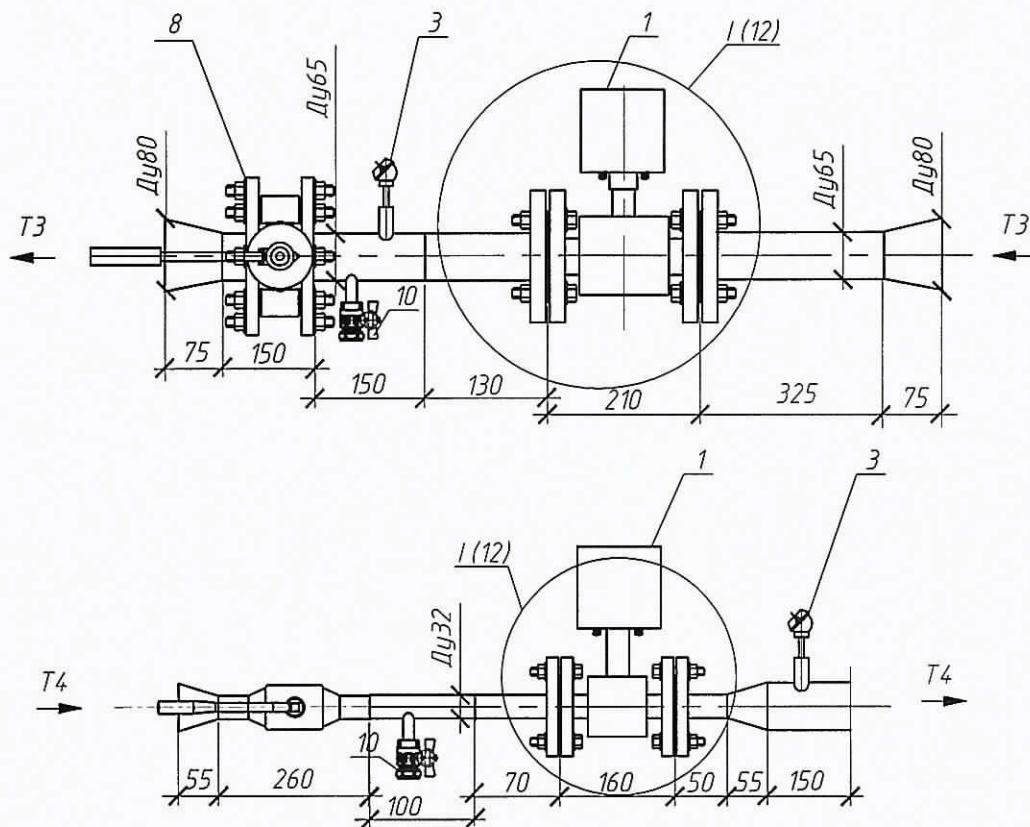
Аксонетрическая схема Т4
