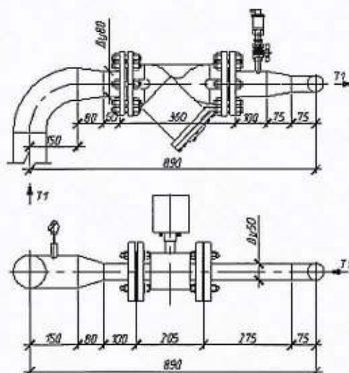
Рисунок 1. Общий вид узла учета
