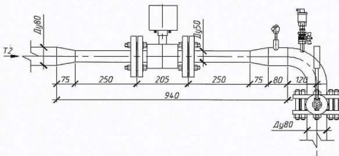
Рисунок 2. Общий вид узла учета
