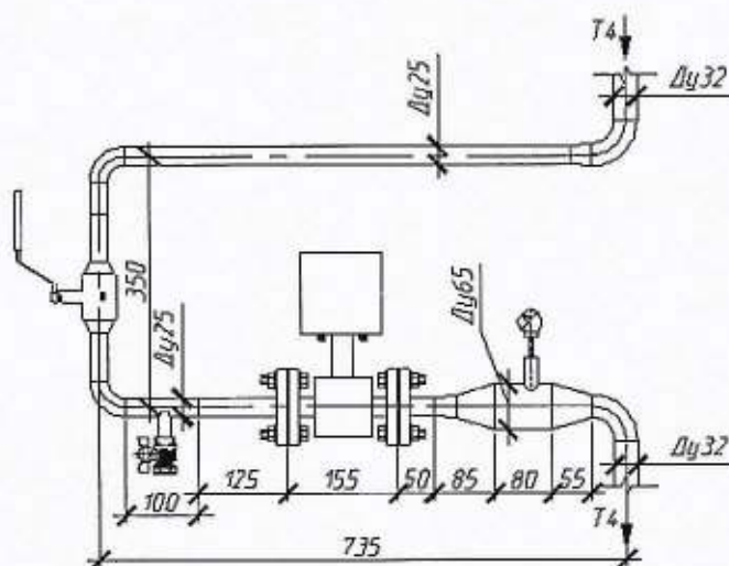
Рисунок 2. Общий вид узла учета
