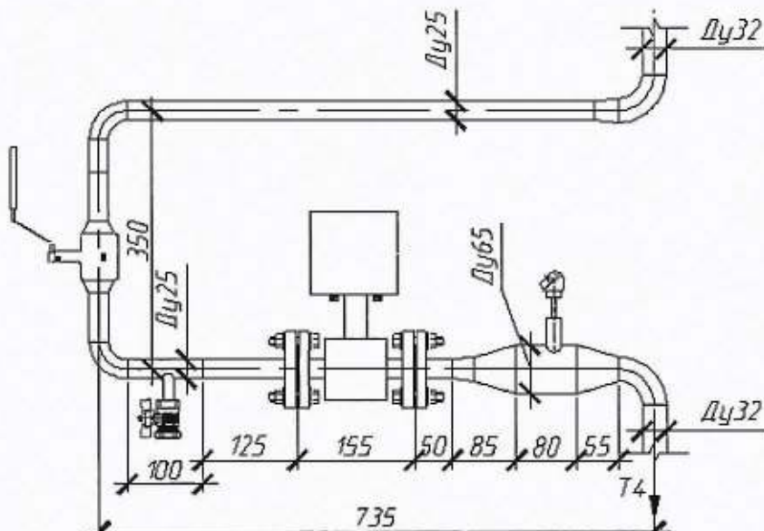
Рисунок 2. Общий вид узла учета
