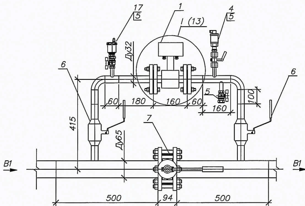
Аксонметрическая схема В1
