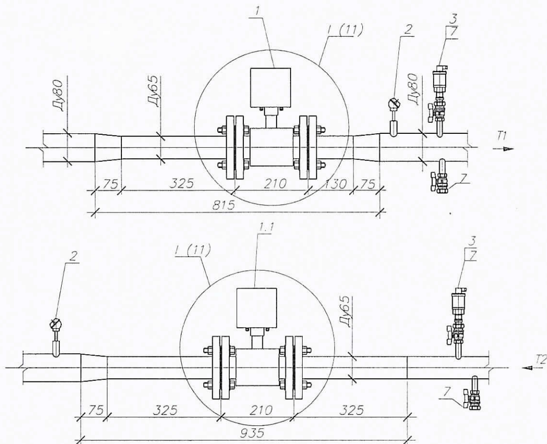
Аксонметрическая схема T2
