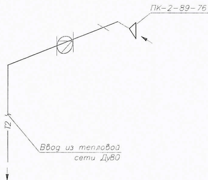
Аксонметрическая схема T2
