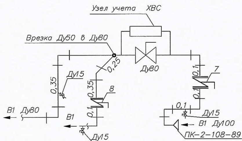
АксонOMETрическая схема B1
