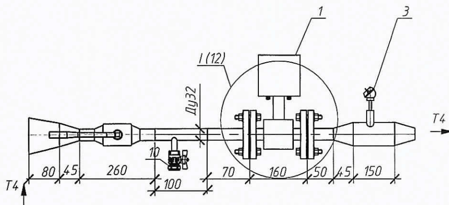
Аксонетрическая схема Т4
