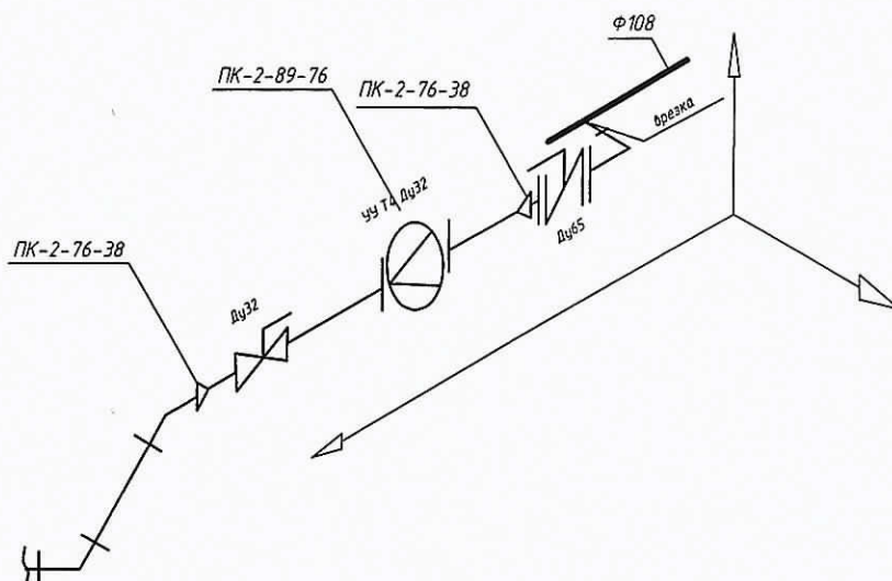
Аксонетрическая схема Т4
