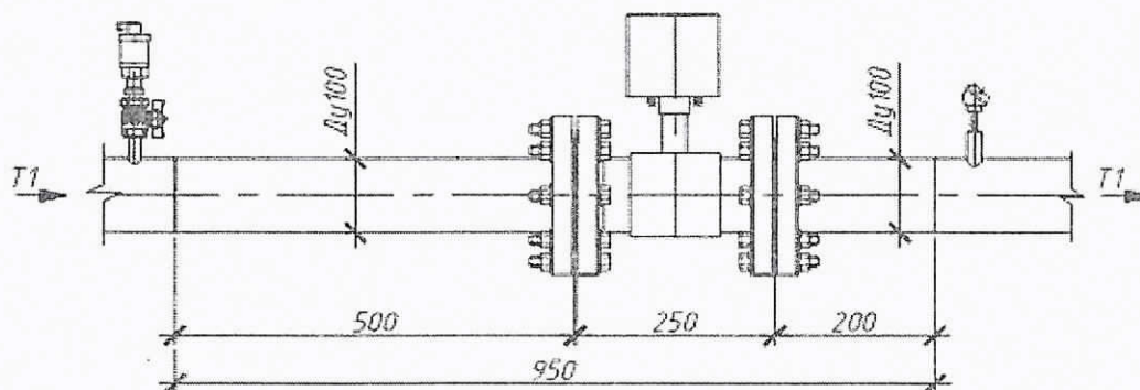
Рисунок 1. Общий вид узла учета
