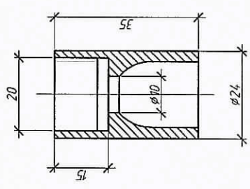
Бобышка термопреобразователя сопротивления
