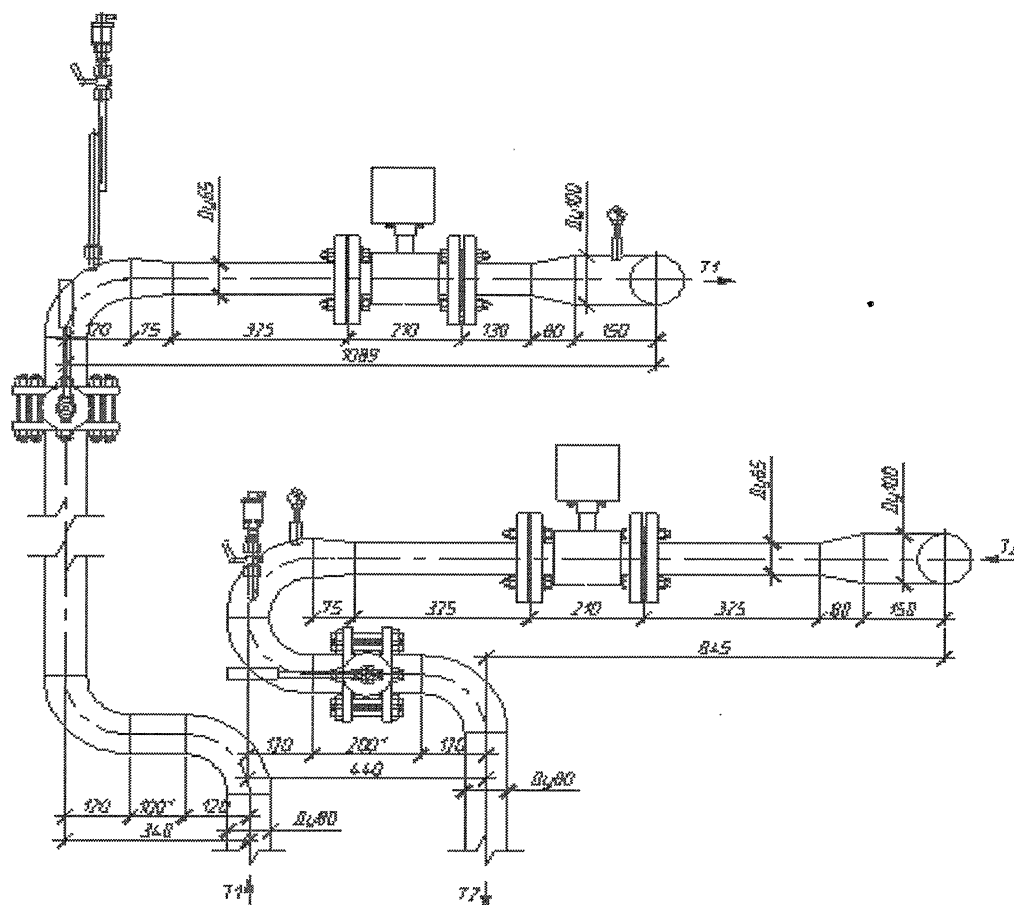
Рисунок 1. Общий вид узла учета
