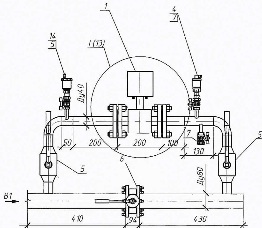
АксонOMETрическая схема В1
