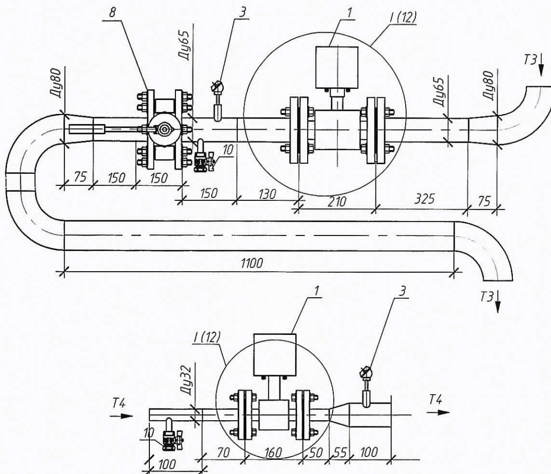
Аксонетрическая схема Т4
