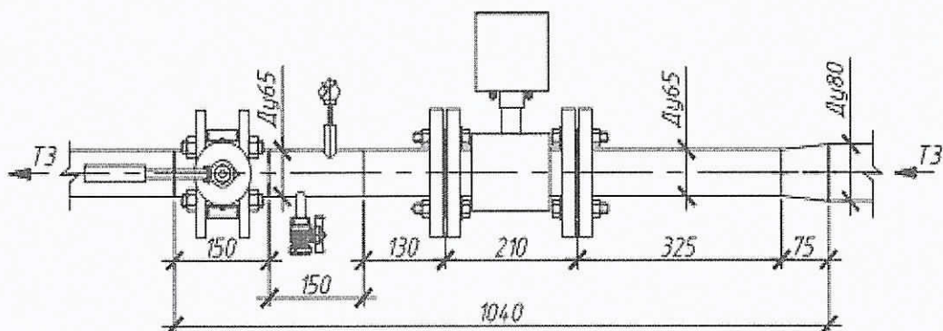
Рисунок 3. Общий вид узла учета
