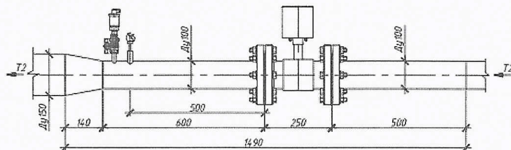
Рисунок 2. Общий вид узла учета
