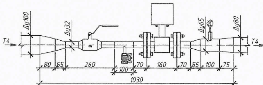
Рисунок 4. Общий вид узла учета
