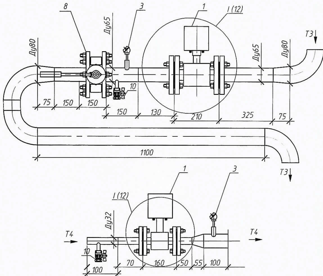
Аксонетрическая схема Т4
