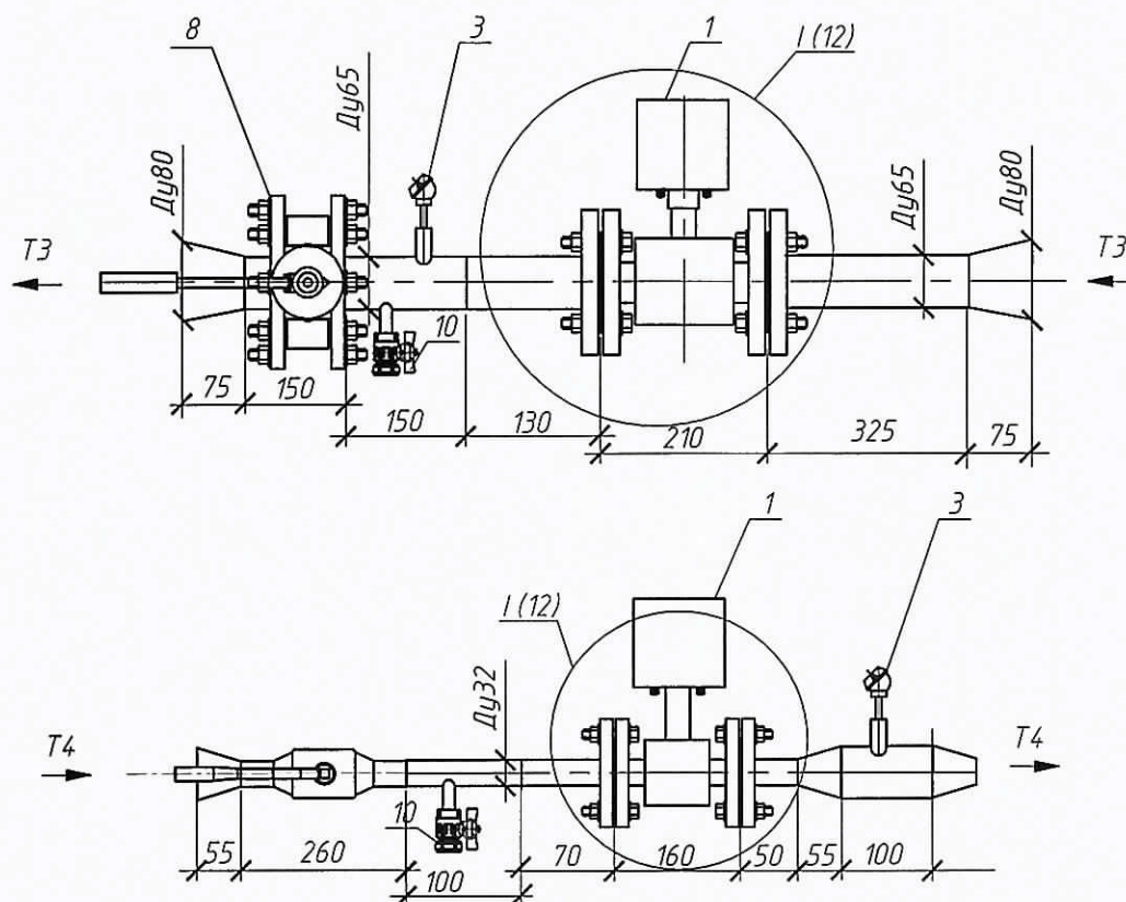
АксонOMETрическая схема Т4
