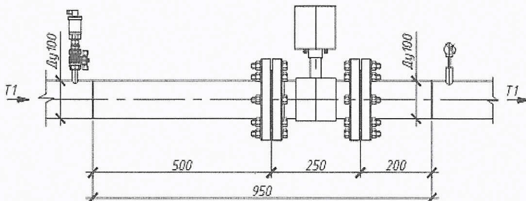
Рисунок 1. Общий вид узла учета
