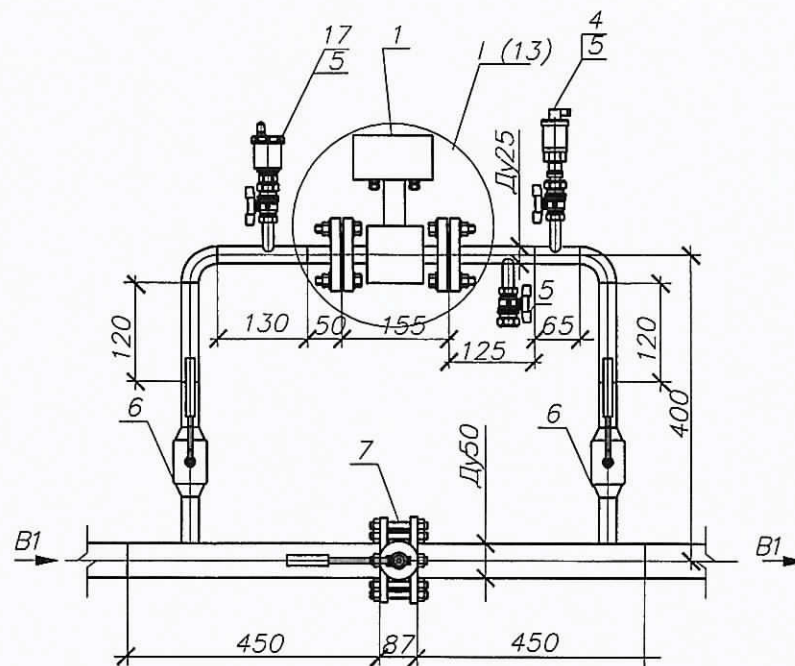
Аксонметрическая схема В1
