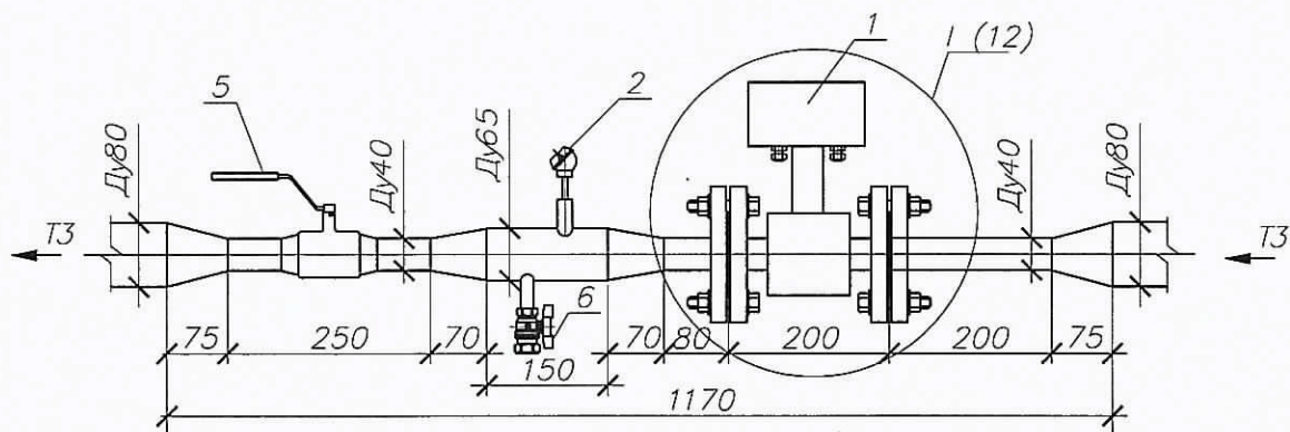
АксонOMETрическая схема ТЗ.
