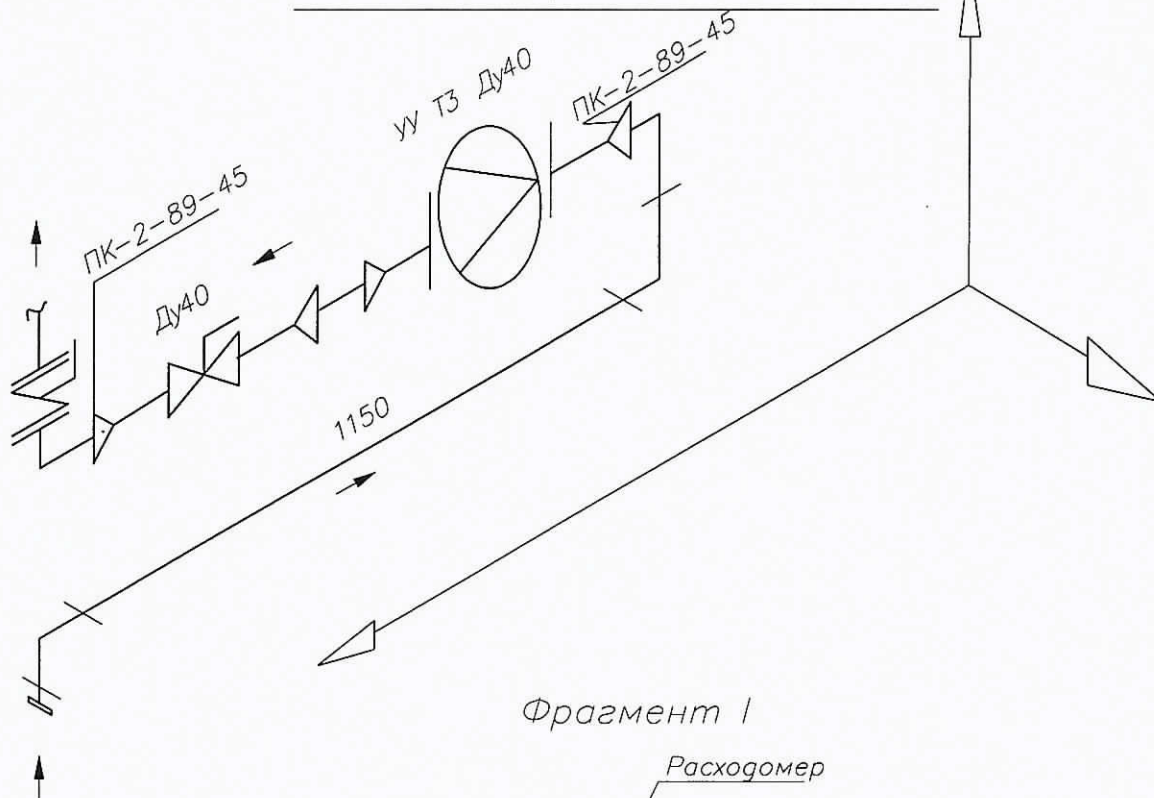
АксонOMETрическая схема ТЗ.
