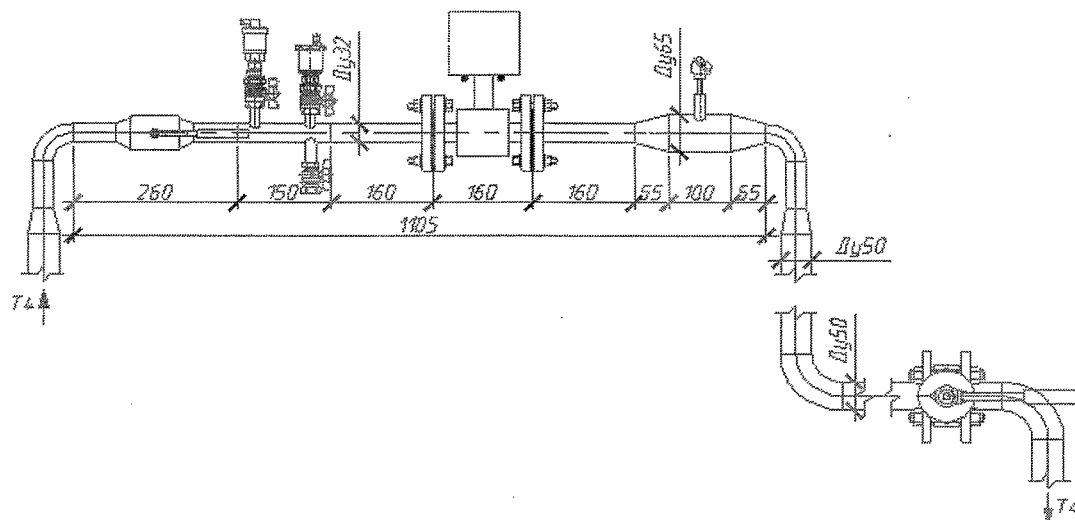
Рисунок 2. Общий вид узла учета
