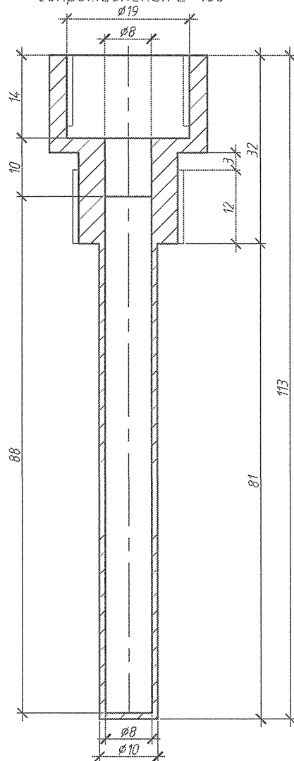
Гильза термопреобразователя сопротивления L=100
