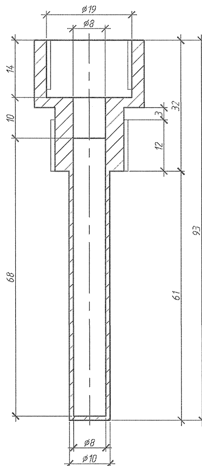
Бобышка термопреобразователя сопротивления
