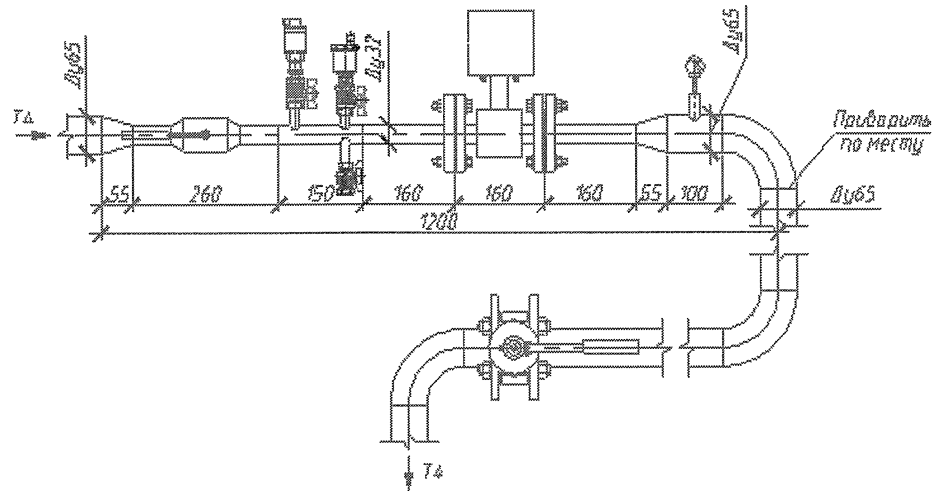
Рисунок 2. Общий вид узла учета
