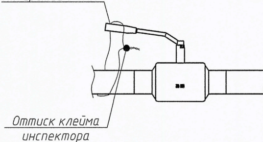
Схема пломбирования шаровых кранов
