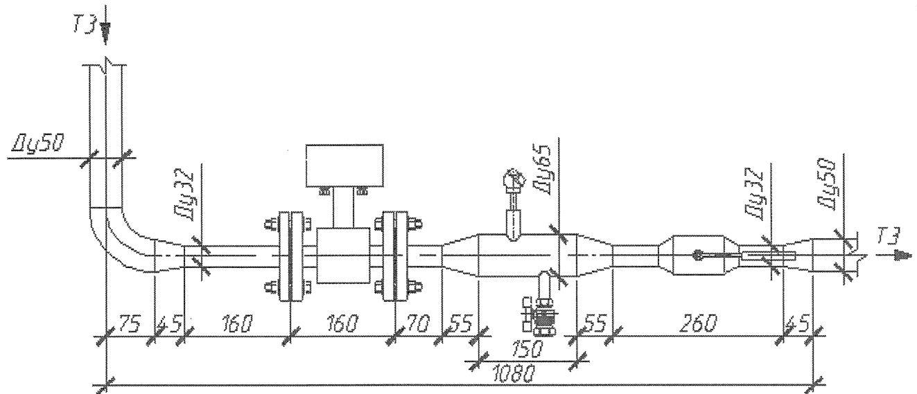
Рисунок 1. Общий вид узла учета
