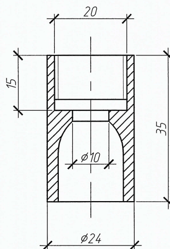
Бобышка термопреобразователя сопротивления
