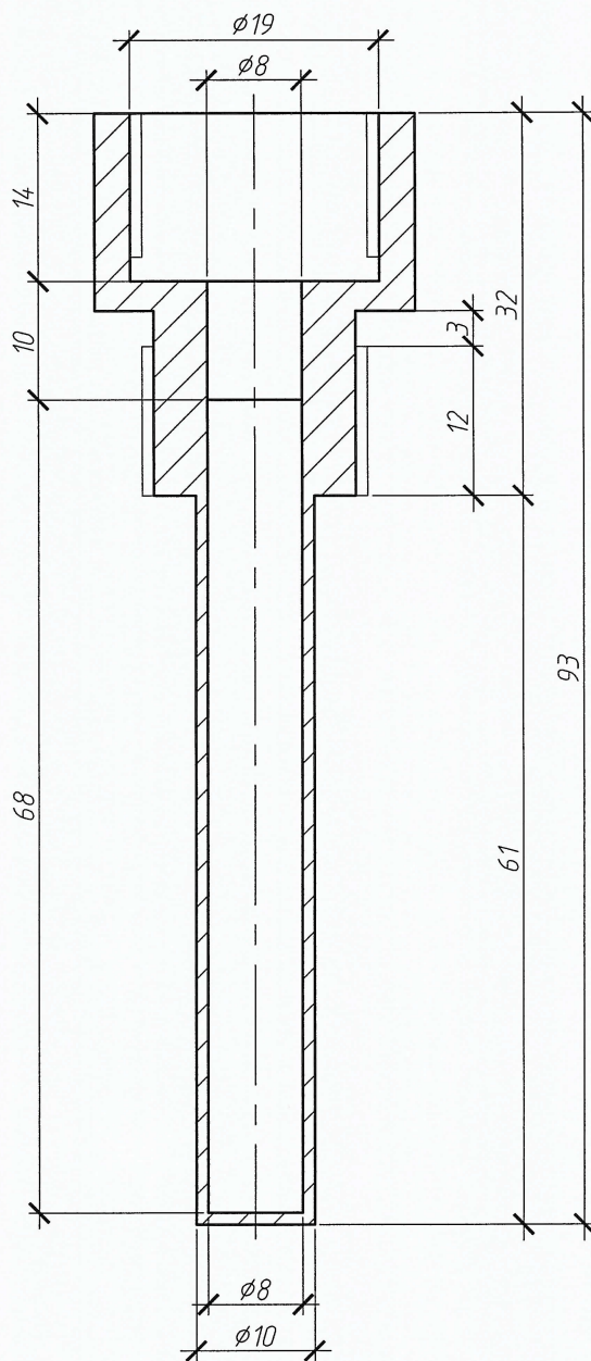
Гильза термопреобразователя сопротивления
