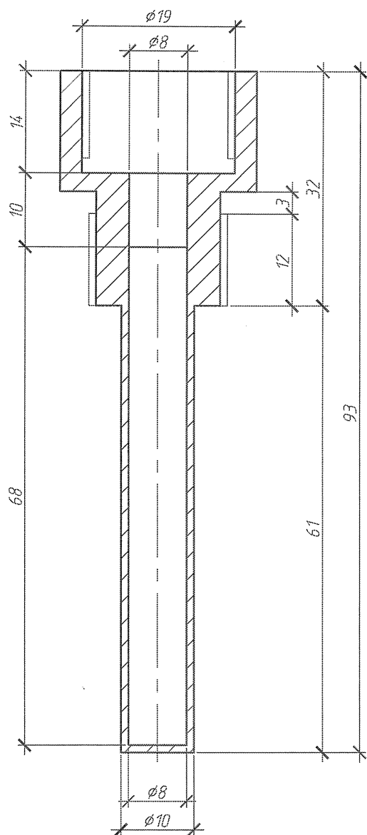
Бобышка термопреобразователя сопротивления
