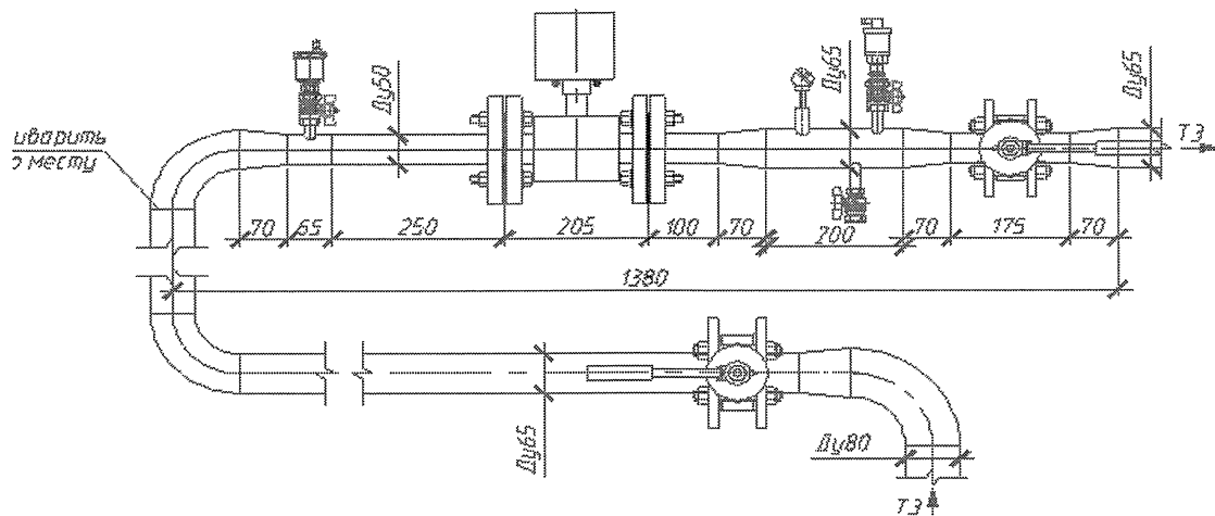
Рисунок 1. Общий вид узла учета
