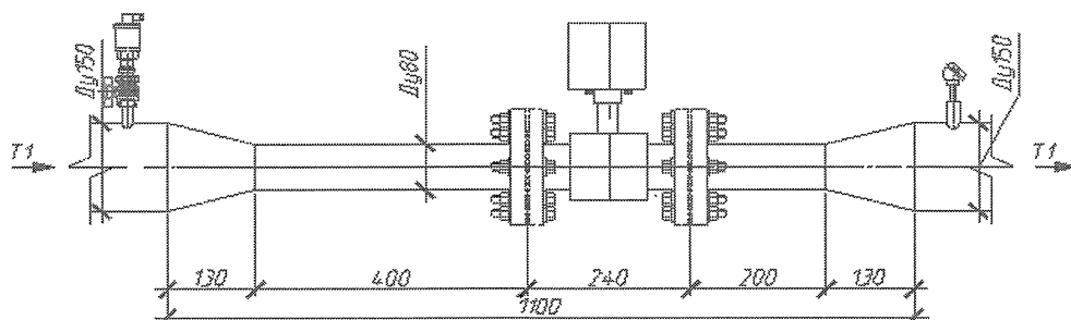
Рисунок 1. Общий вид узла учета
