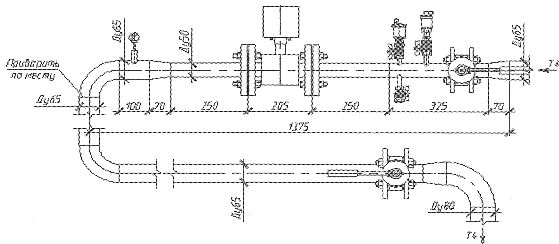
Рисунок 2. Общий вид узла учета
