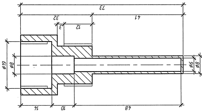
Гильза термопреобразователя сопротивления L=60
