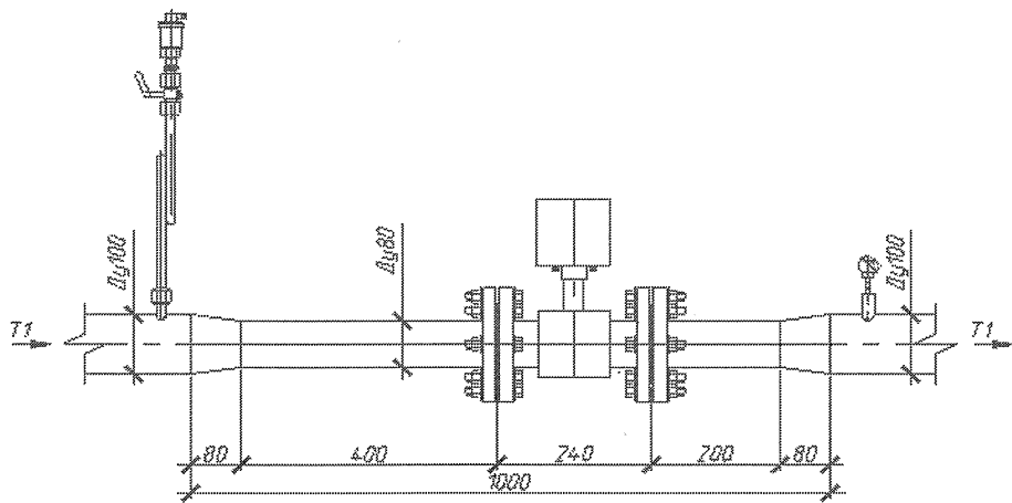
Рисунок 1. Общий вид узла учета
