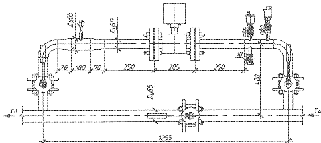
Рисунок 2. Общий вид узла учета
